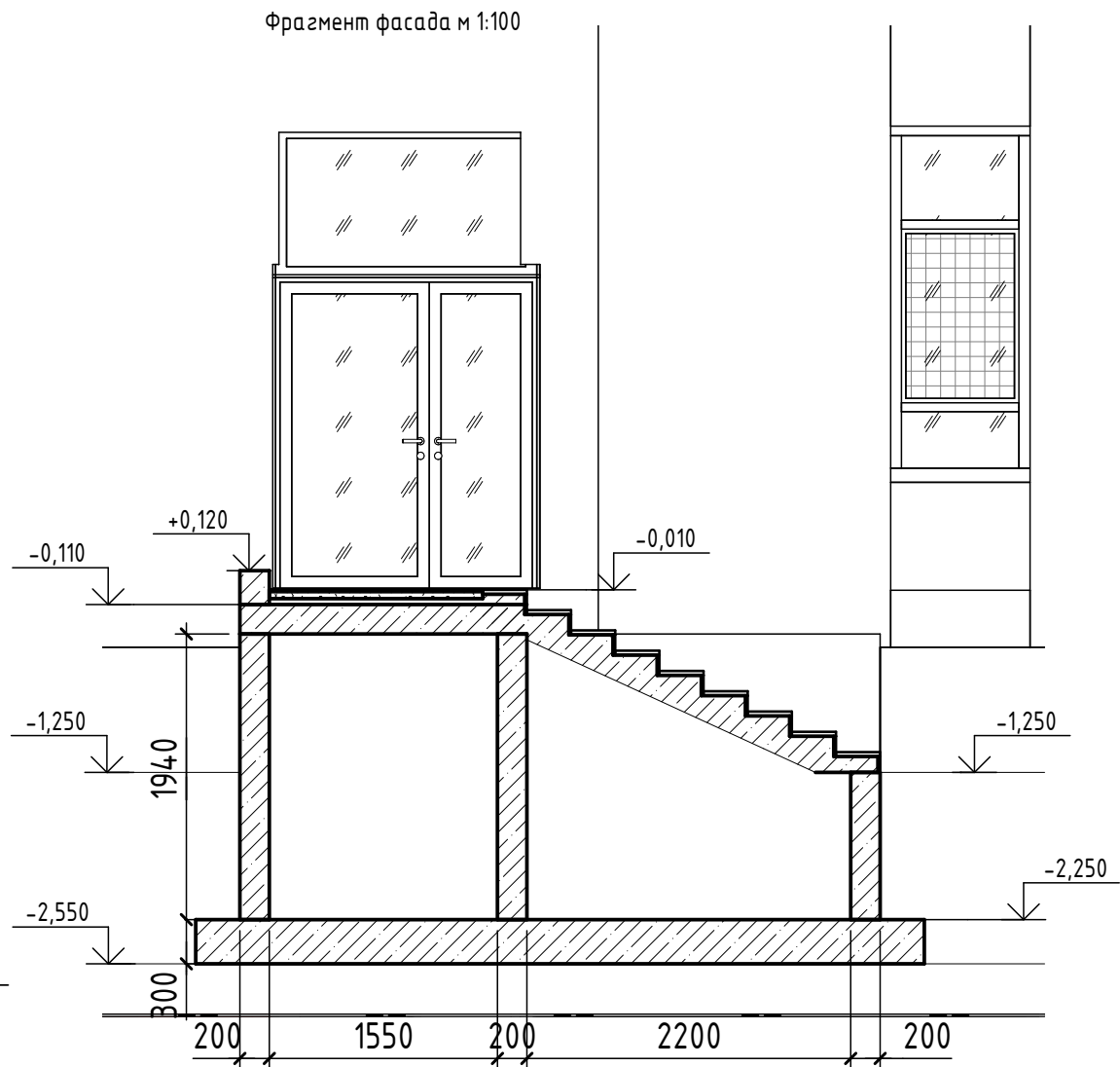
Фрагмент фасада м 1:100
